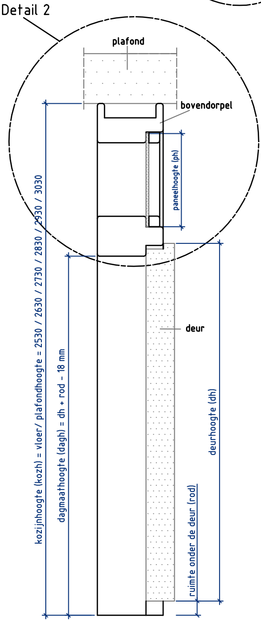
Doorsnede BB
