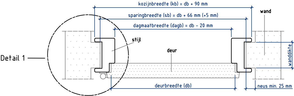
Doorsnede AA
