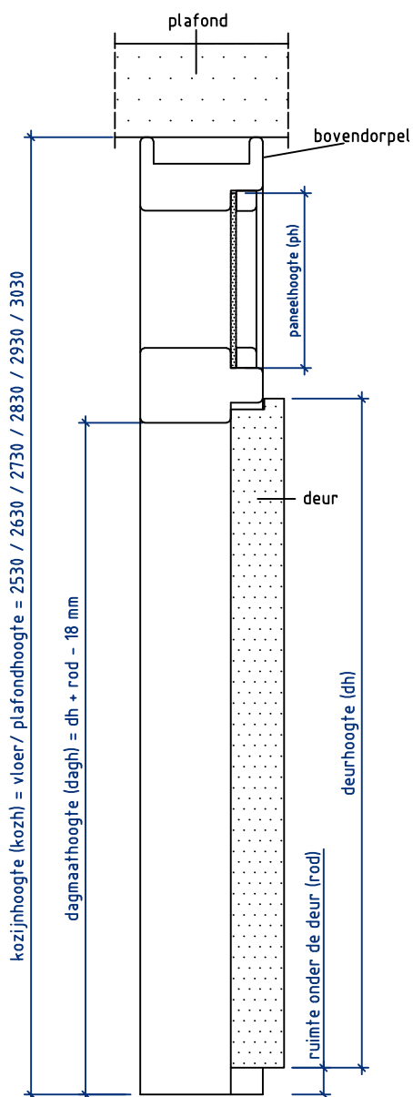
Doorsnede BB
