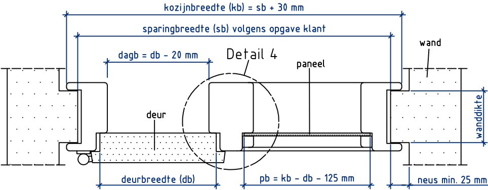
Doorsnede AA
