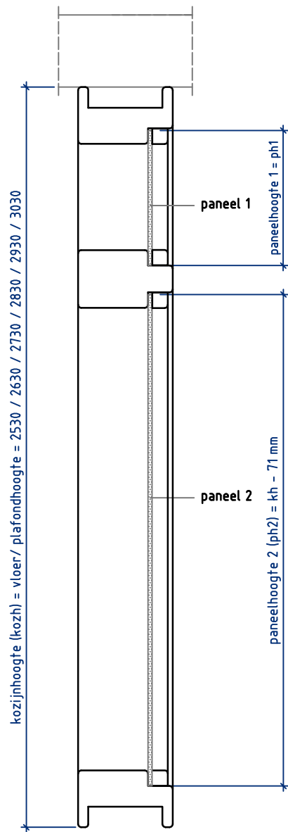
Doorsnede CC
