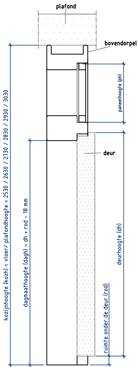
Doorsnede BB
