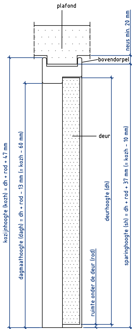
Doorsnede BB
