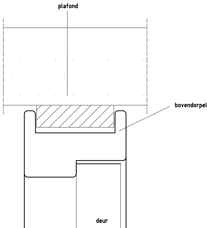
Detail 2: bovendorpel
