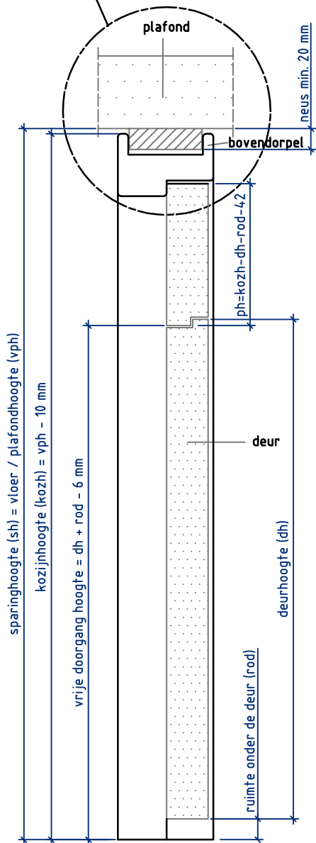
Doorsnede BB
