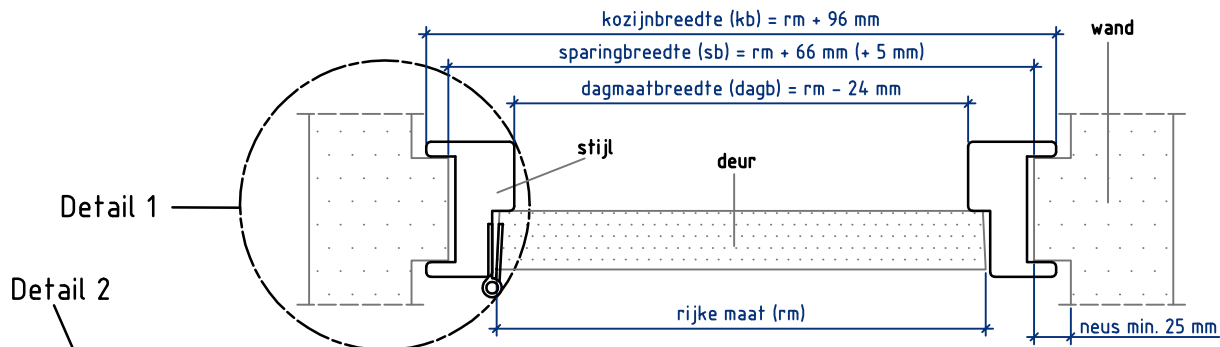
Doorsnede AA
