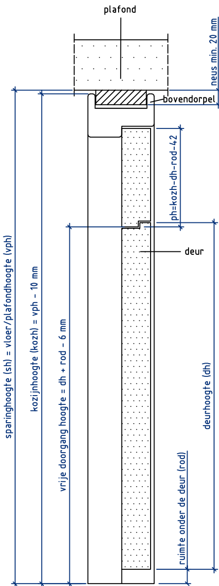
Doorsnede BB
