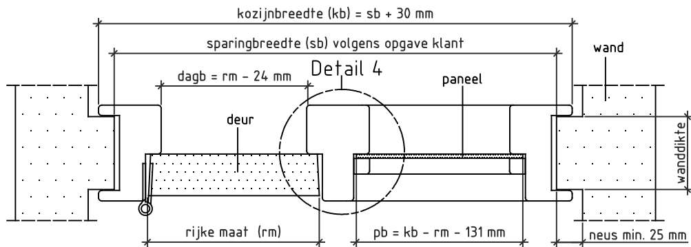
Doorsnede AA
