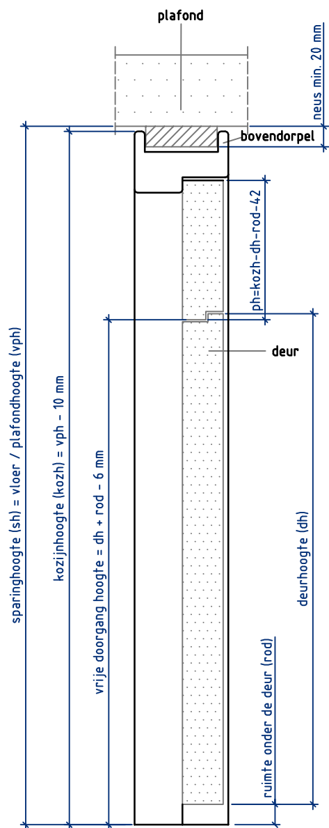
Doorsnede BB
