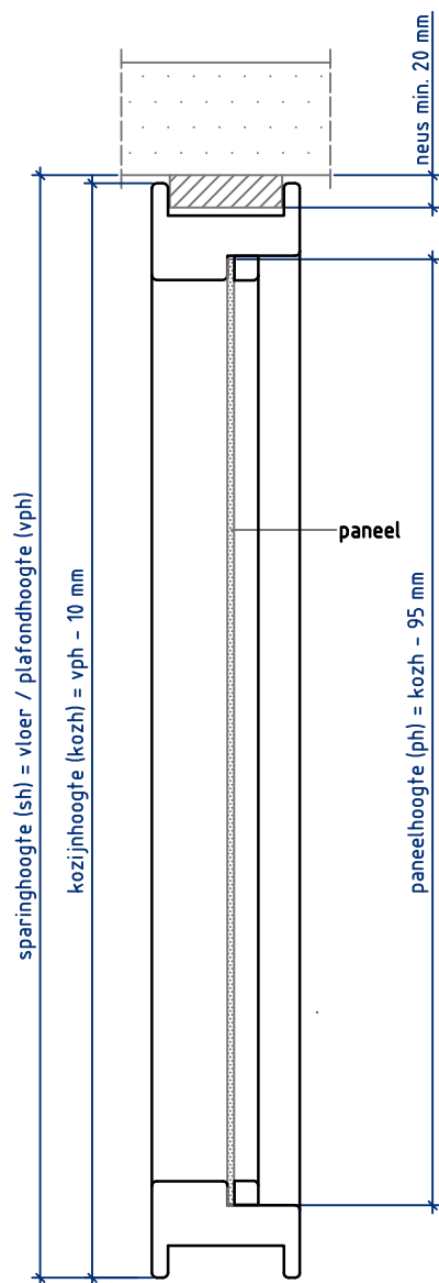
Doorsnede CC
