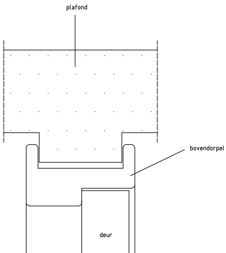
Detail 2: bovendorpel
