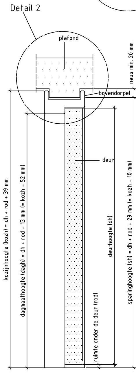
Doorsnede BB
