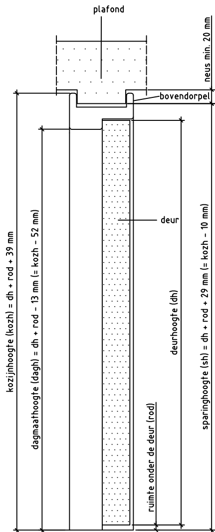
Doorsnede BB
