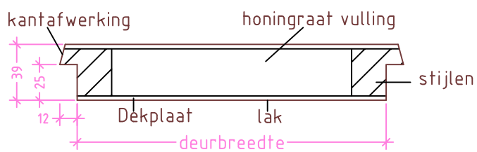
Doorsnede AA
