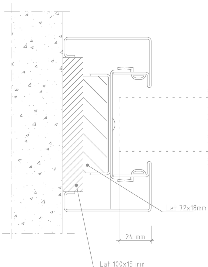
Afb. 2 Aansluiting bij haakse wand, toepassing extra lat 100/125* x 15 mm.
