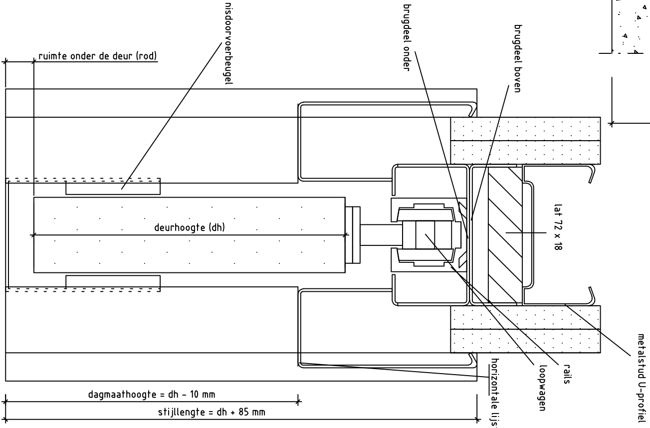
Doorsnede AA
