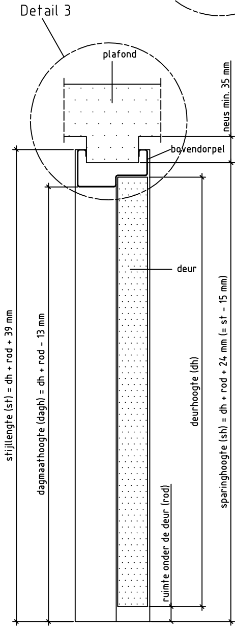
Doorsnede BB
