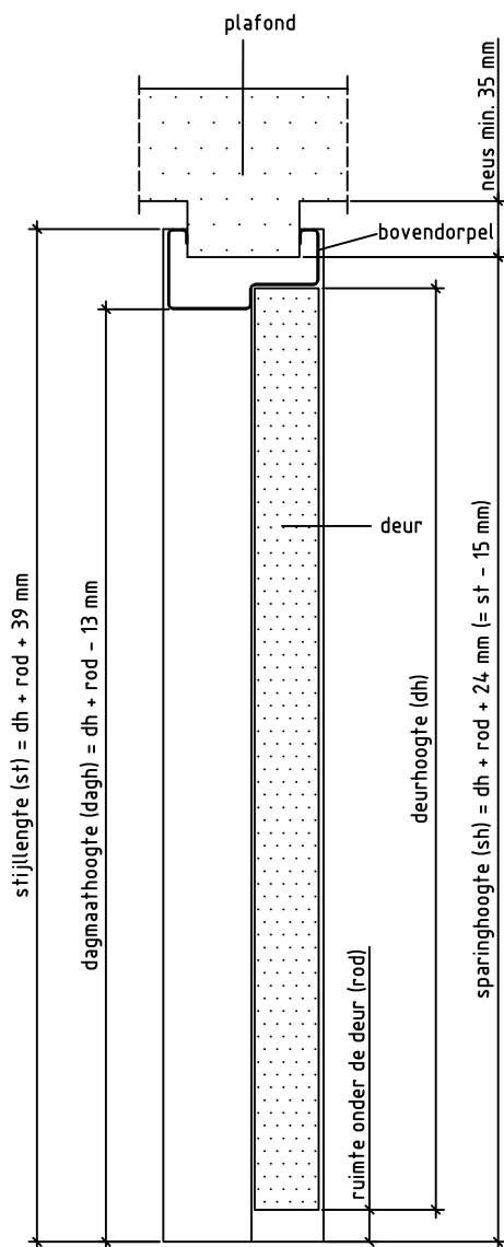
Doorsnede BB
