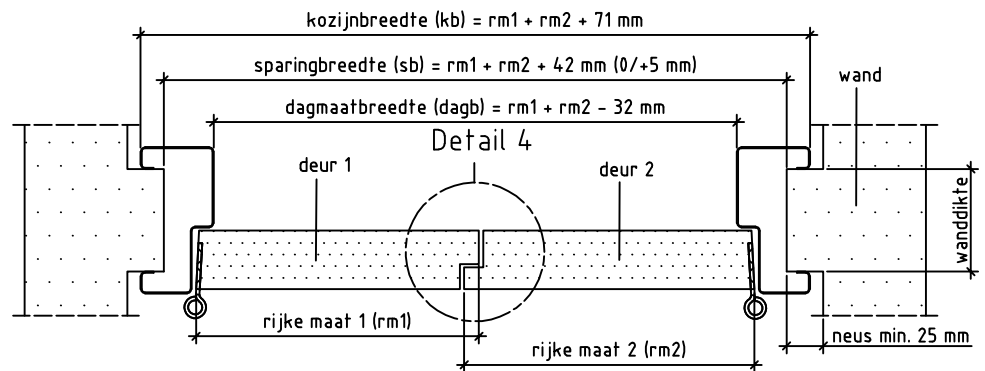
Doorsnede AA
