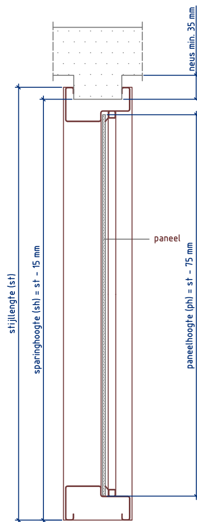
Doorsnede CC
