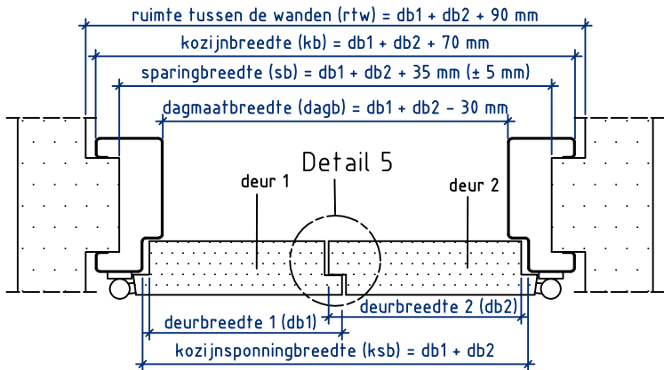
Doorsnede AA sponning/contrasponning
