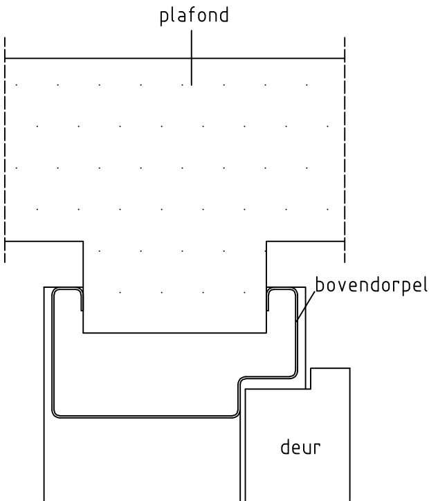
Detail 3: bovendorpel
