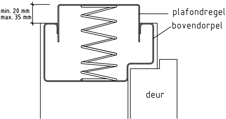
Detail 4: Optioneel plafondregel
