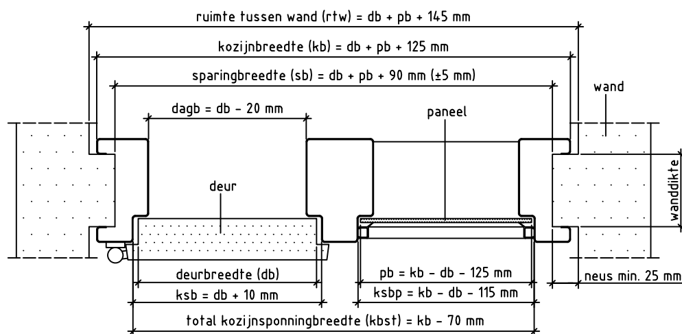
Doorsnede AA
