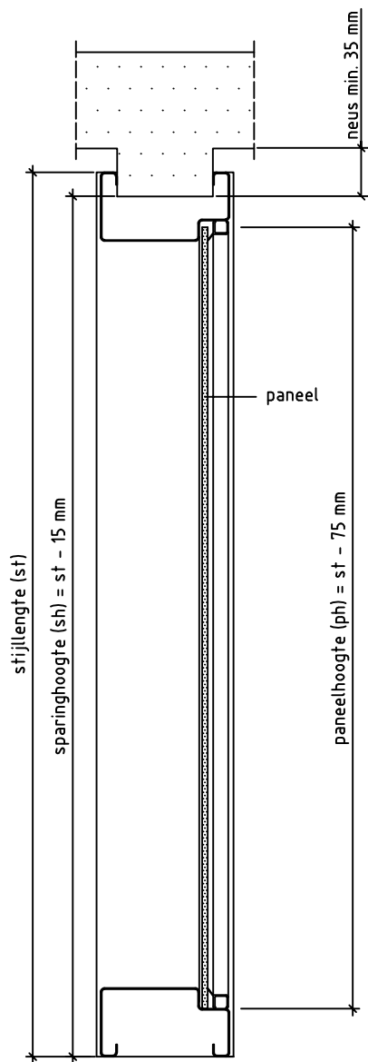
Doorsnede CC
