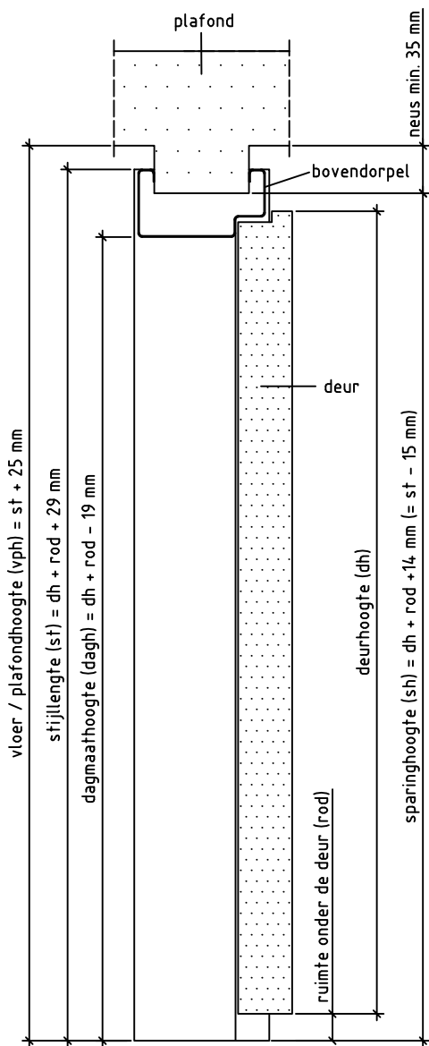
Doorsnede BB
