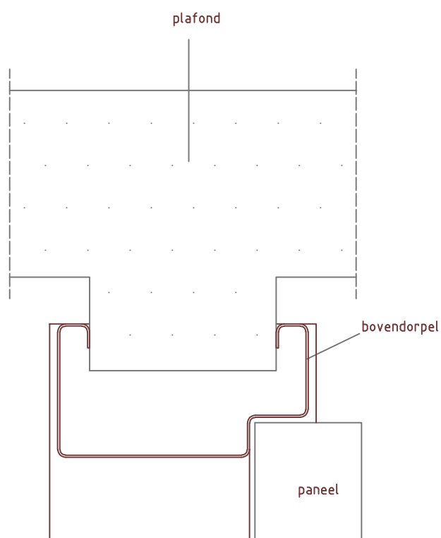
Detail 4: Optioneel plafondregel
