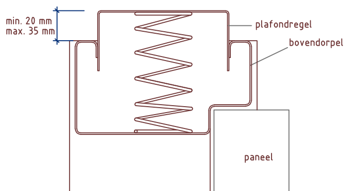
Detail 4: Optioneel plafondregel
