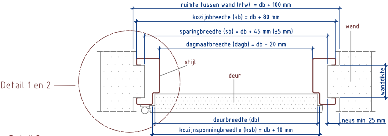
Doorsnede AA
