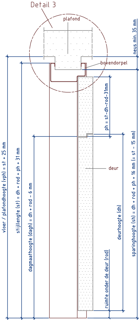
Doorsnede BB
