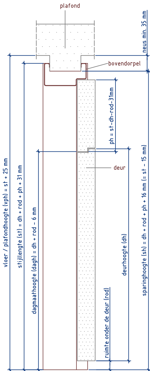
Doorsnede BB
