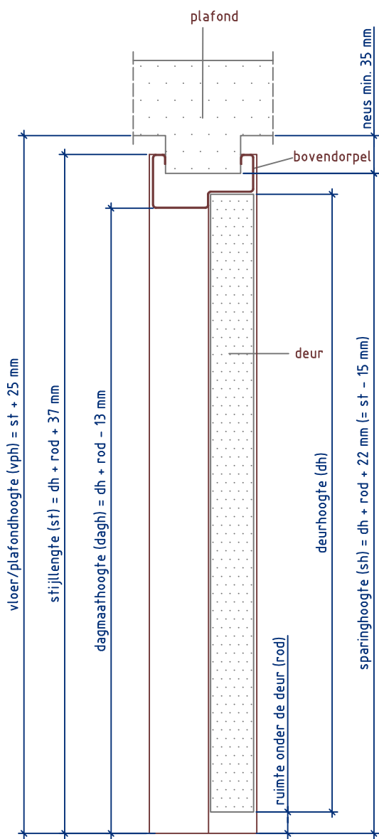
Doorsnede BB
