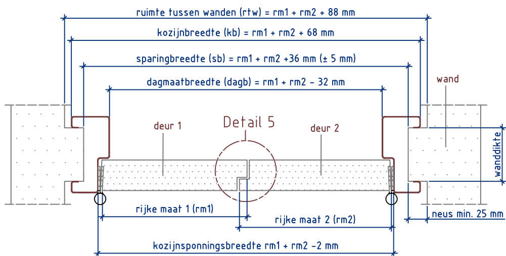
Doorsnede AA
