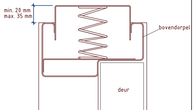
Detail 4: optionele plafondregel
