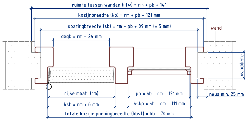
Doorsnede AA
