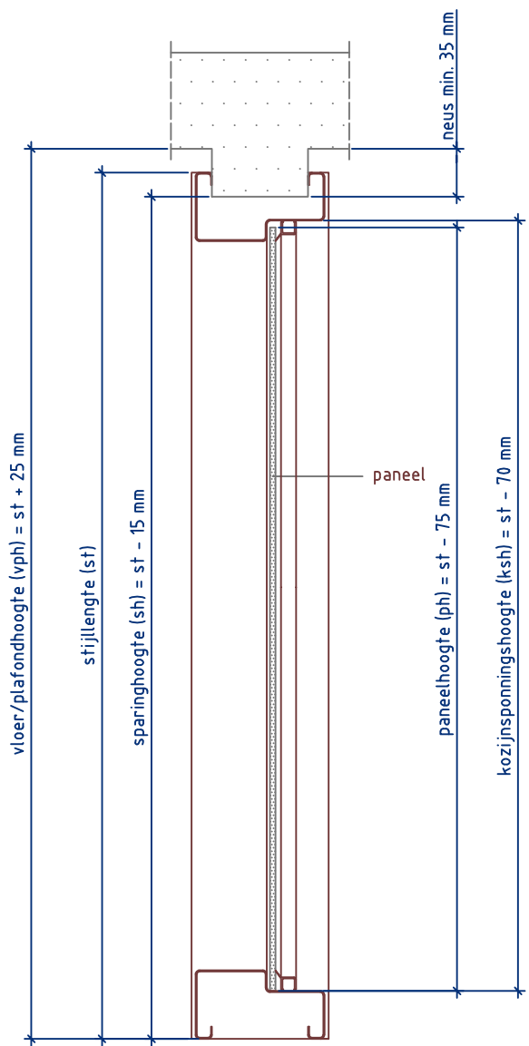
Doorsnede CC
