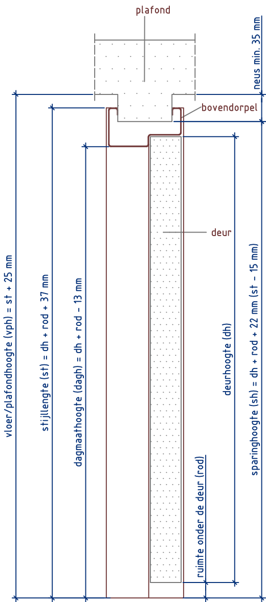
Doorsnede BB
