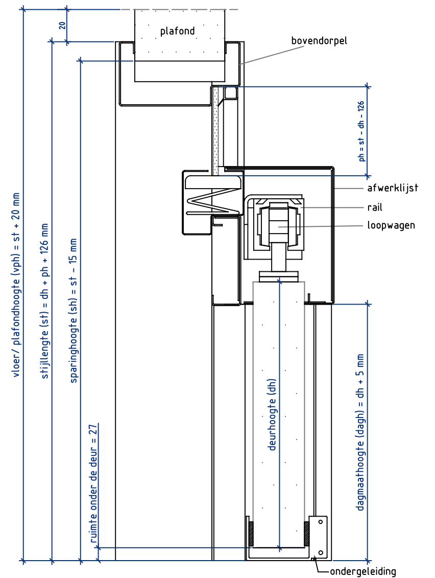
Doorsnede CC
