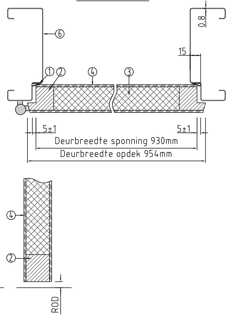
Doorsnede BB
