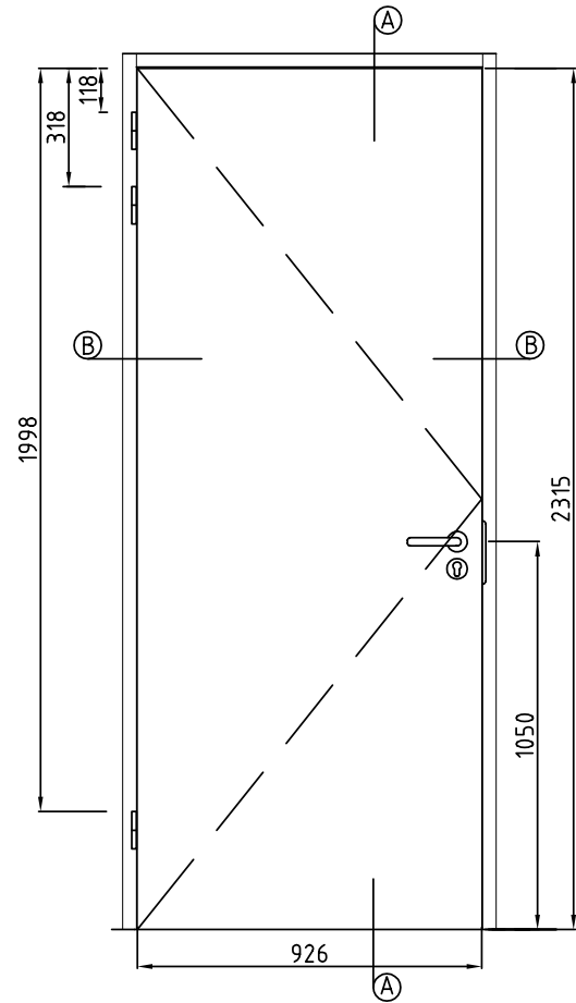
Vooraanzicht
