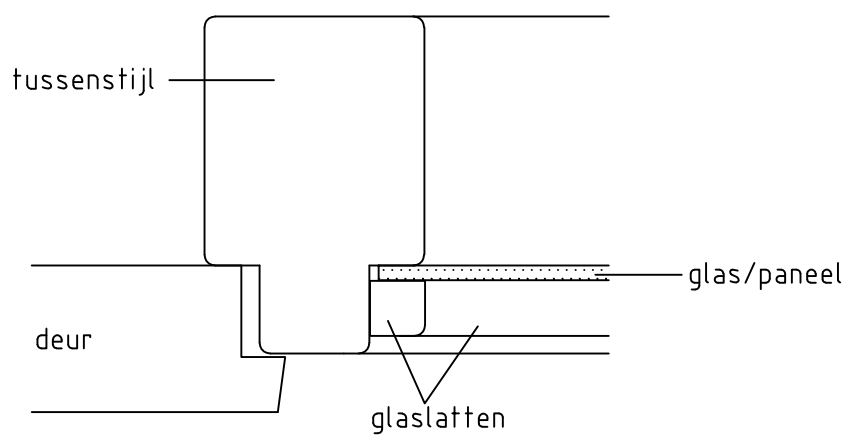
Detail 4: tussenstijl
