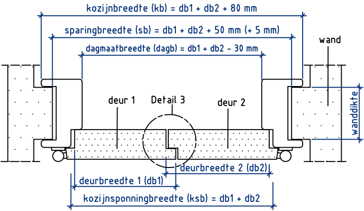
Doorsnede AA sponning/contrasponning
