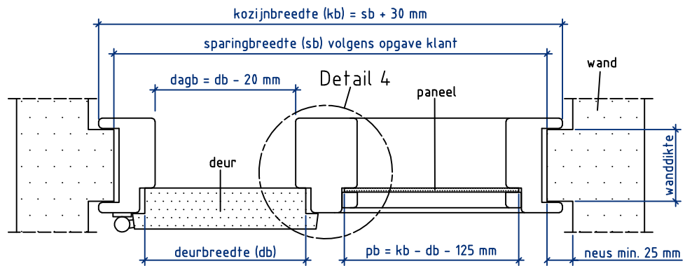
Doorsnede AA
