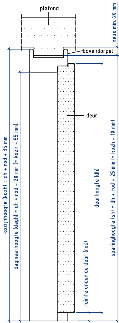
Doorsnede BB
