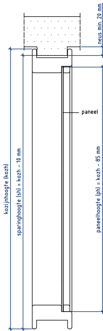
Doorsnede CC
