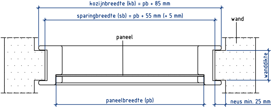
Doorsnede AA
