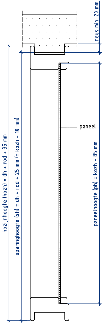
Doorsnede BB
