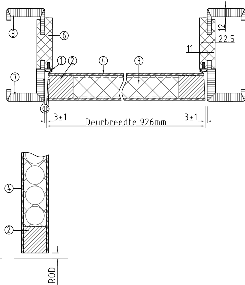
Doorsnede BB
