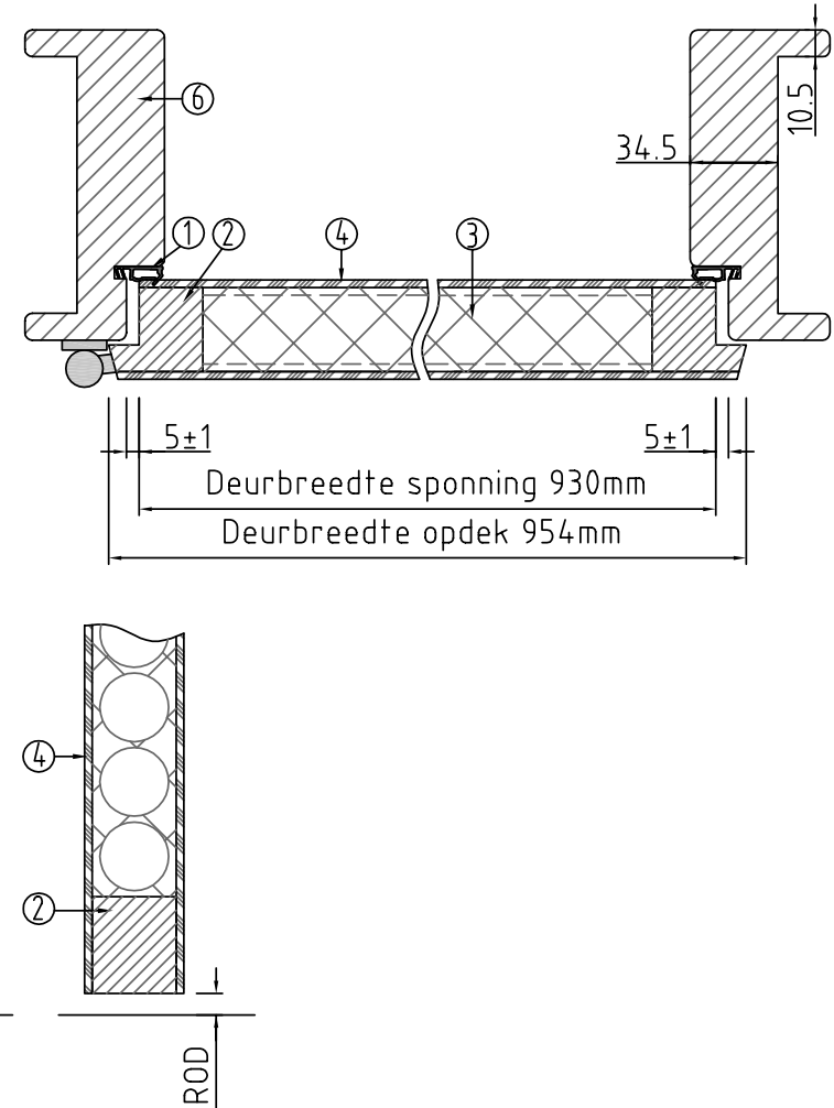
Doorsnede BB
