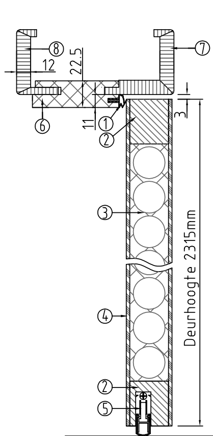
Doorsnede AA
