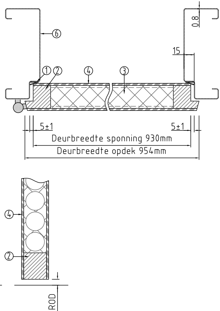
Doorsnede BB
