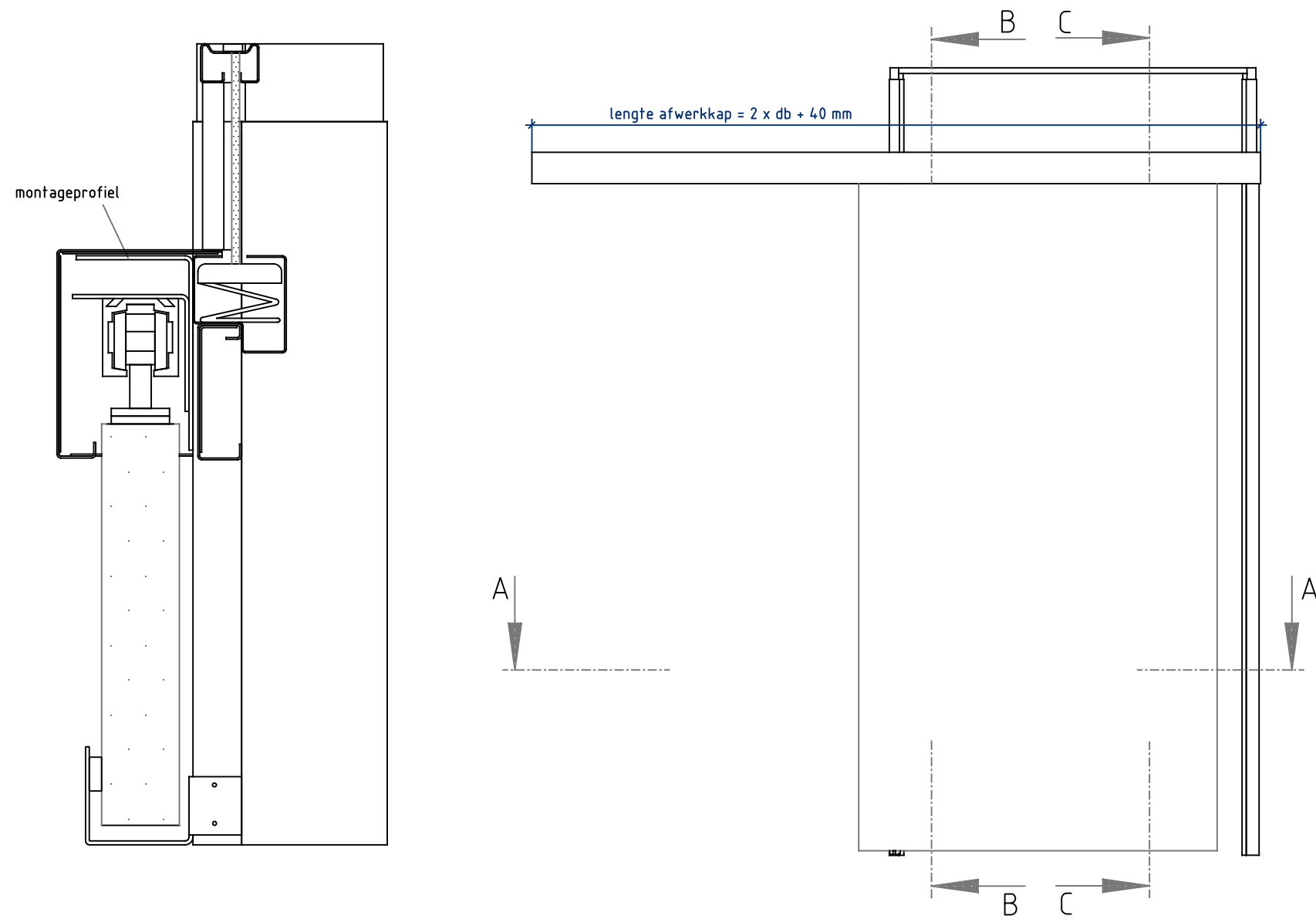
Doorsnede BB
