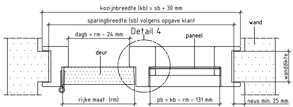
Doorsnede AA
