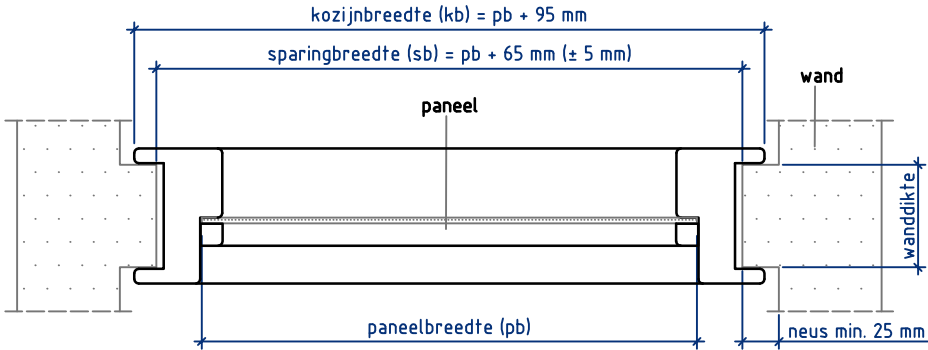
Doorsnede AA
