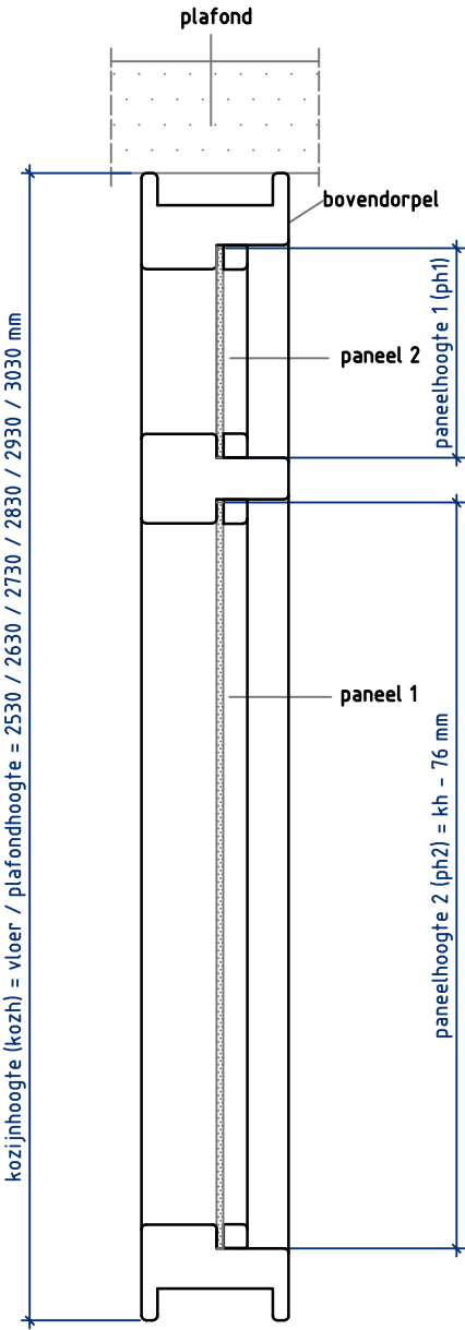
Doorsnede BB
