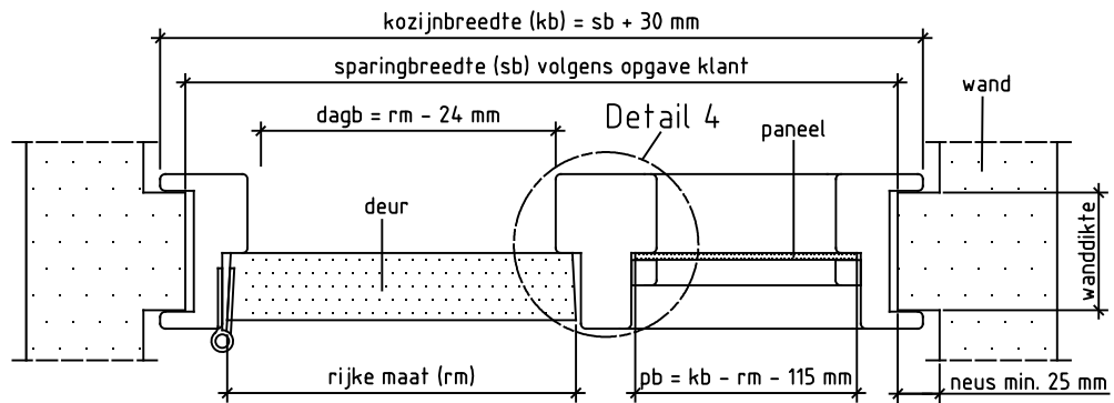
Doorsnede AA
