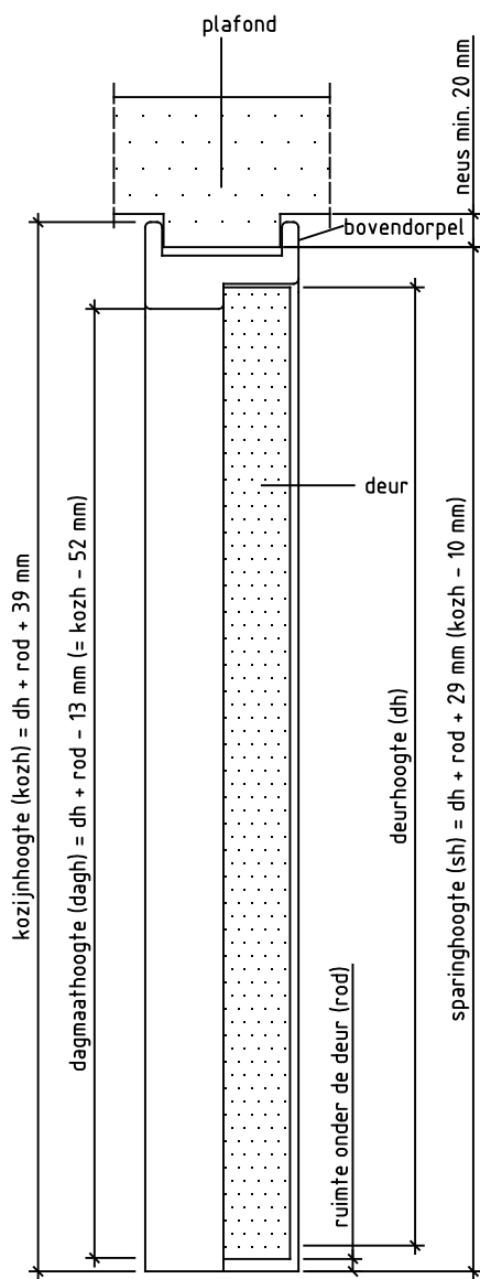
Doorsnede BB
