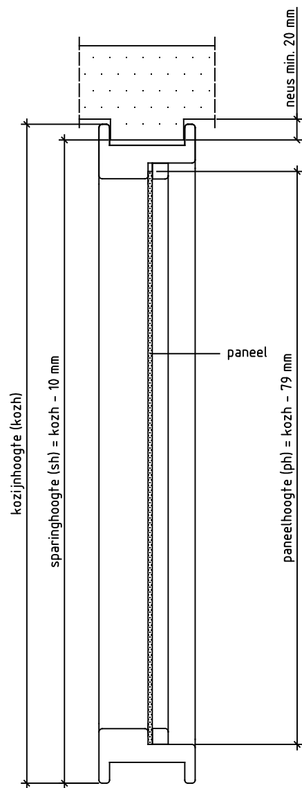
Doorsnede CC
