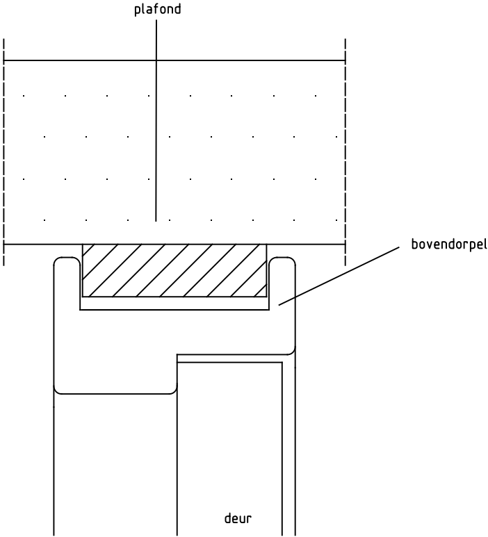
Detail 2: bovendorpel
