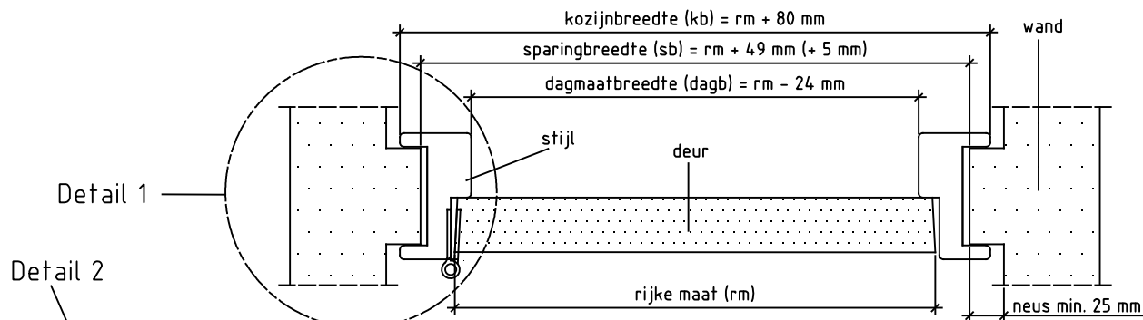
Doorsnede AA
