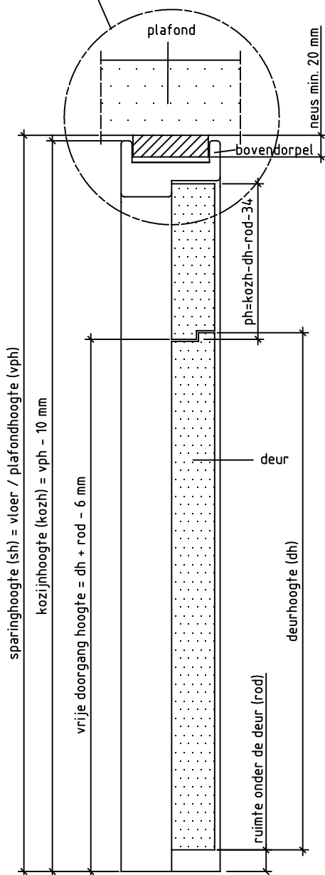
Doorsnede BB
