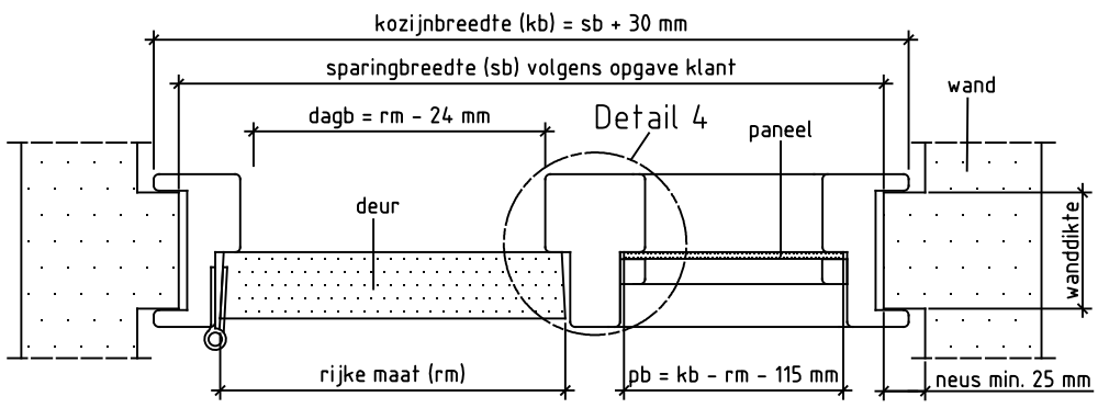
Doorsnede AA
