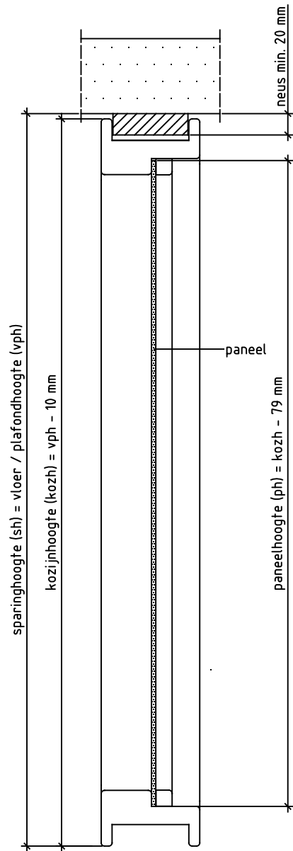
Doorsnede CC
