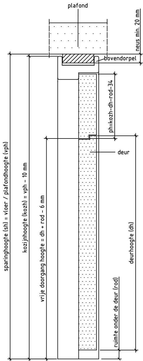
Doorsnede BB
