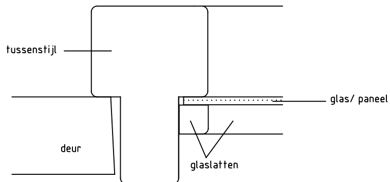
Detail 4: tussenstijl
