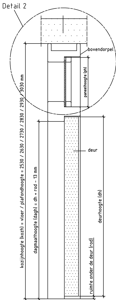
Doorsnede BB
