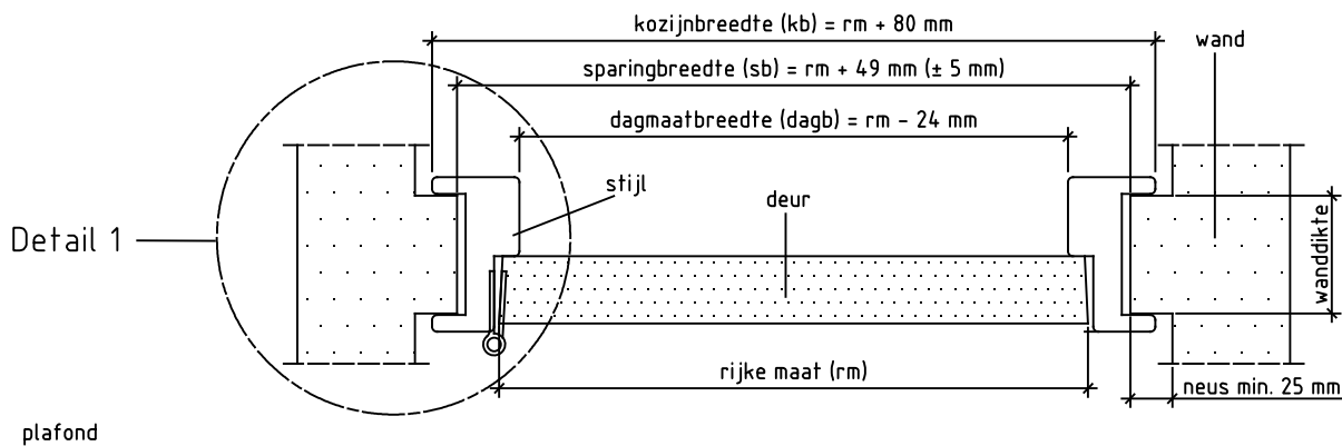
Doorsnede AA
