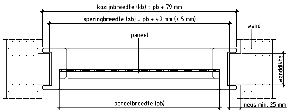
Doorsnede AA
