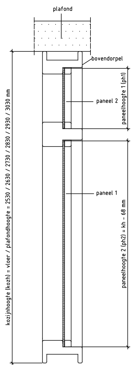
Doorsnede BB
